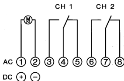
Wiring schematic
